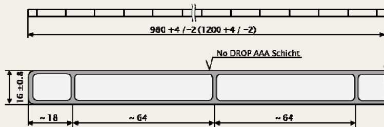
Querschnitt der PLEXIGLAS® Heatstop Cool Blue AAA SDP 16-64 (Maße in mm)
