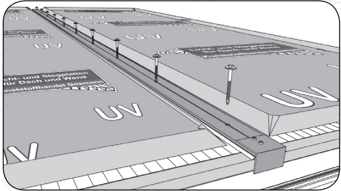
VA-Schraube, 70 mm mit Neoprendichtung
